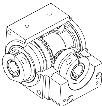
RAH(空心軸)
