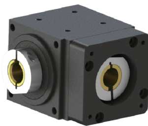
RAH(空心軸)
