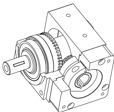
RAS(實心軸)
